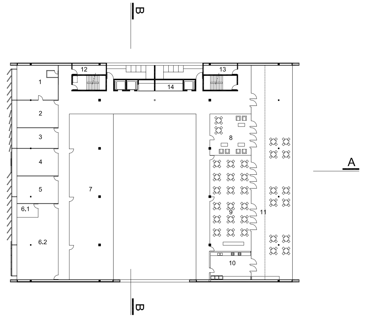
PLANTA 2º PAVIMENTO
