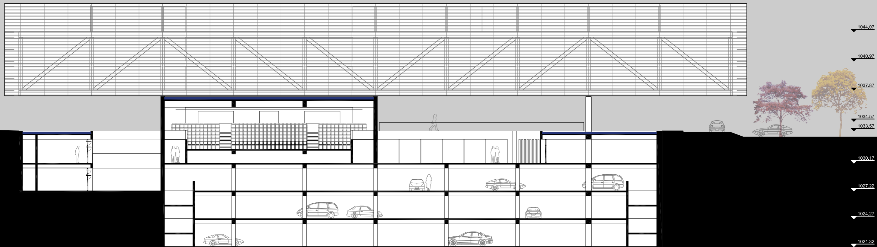
CORTE AA_esc: 1/250
