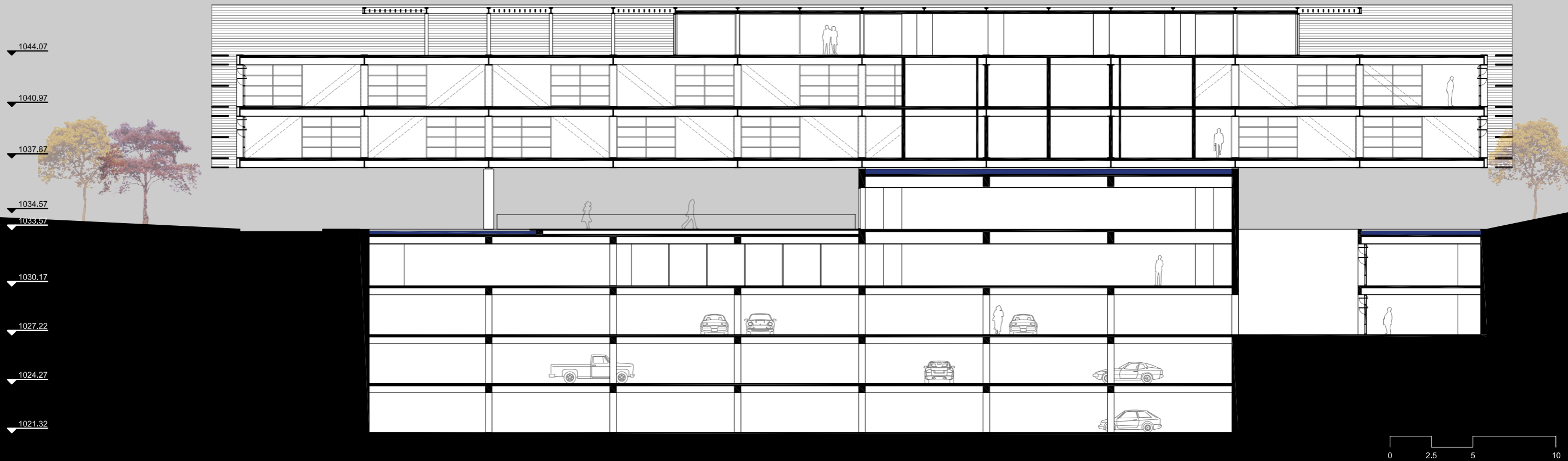
CORTE BB_esc: 1/250
